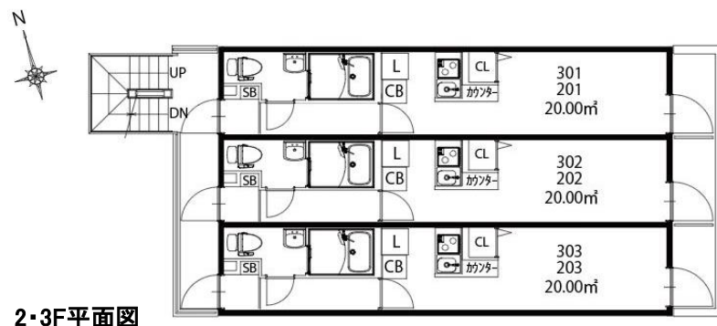
2・3F平面図
