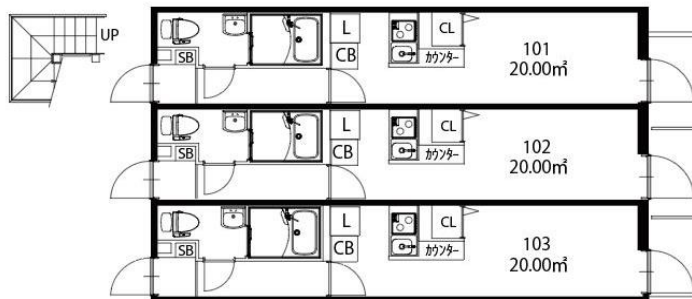
1F平面図
